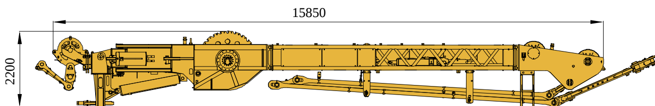
超起装置 34 t Super lifting device
