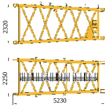
大小加长节 4.7/4.3 t Extensions
