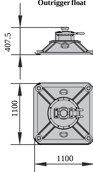
支脚垫板 3.731 t Outrigger pad
